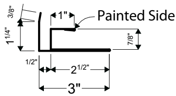
16B | MINI FJTRIM
