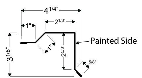
06B | MINI MINI GABLE
