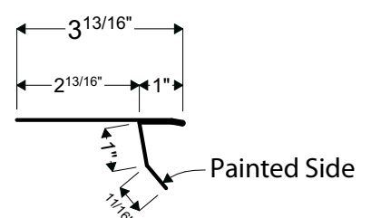
09B | DRIP EDGE B
