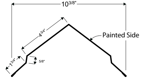
01C | RIDGE CAP (OVERSIZE 10/12)
