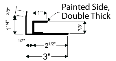
16D | FULL WRAP MINI FJTRIM
