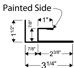
16 | FJTRIM
