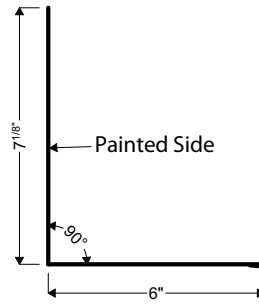
04E | SIDEWALL
