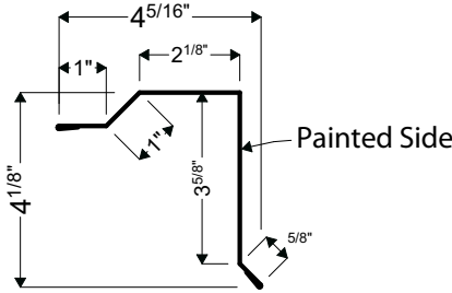
06 | MINI GABLE
