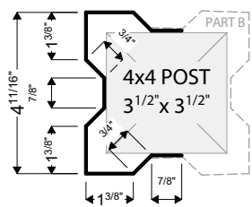
304A, 304B | 4x4 POST WRAP
