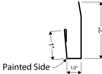
05B | MINI J-CHANNEL
