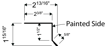
09 | DRIP EDGE
