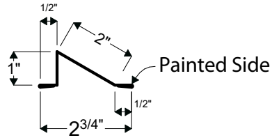
12B | MINI SNOW GUARD
