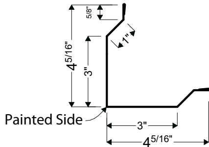
14C | MINI OUTSIDE CORNER
